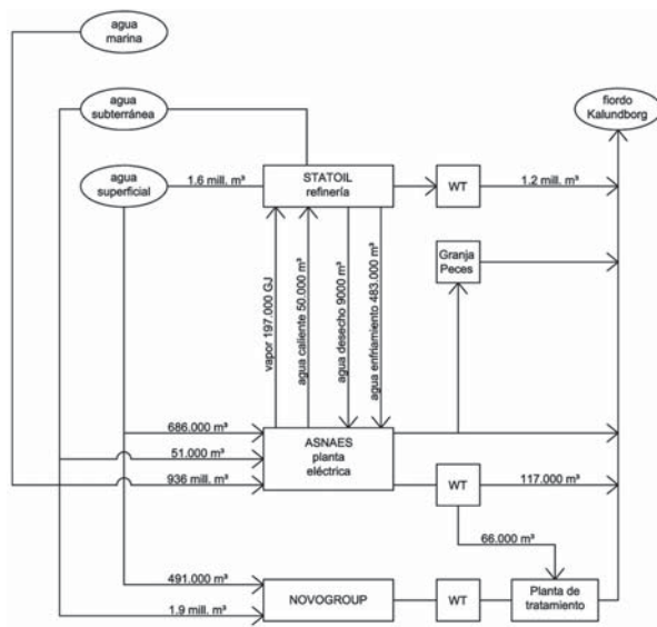
Figura 3: Simbiosis Industrial del flujo de agua en Kalundborg (m 3 /año) en 2002. Fuente: Green Accounts from Kalundborg Center for Industrial Symbiosis (Hansen 2004). El estudio de SFA (Análisis de Flujo de Sustancia) del agua en Kalundborg parte de medir y rastrear la magnitud de las presiones humanas sobre las funciones ambientales. Para luego identificar las conexiones entre las demandas y las actividades económicas y generar los datos requeridos para monitorear las políticas ambientales de reducción de metabolismo
