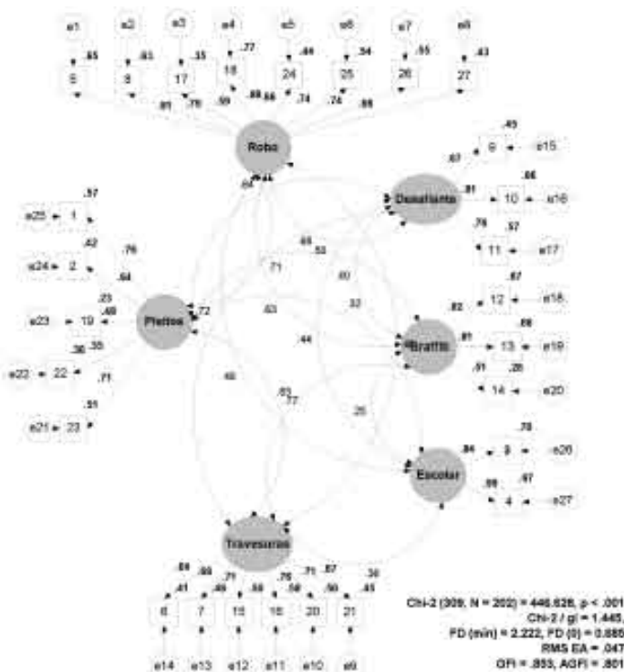
Figura 2. Parámetros estandarizados del modelo de seis factores correlacionados con los 27 ítems originales (estimados por Mínimos Cuadrados Generalizados, GLS).
