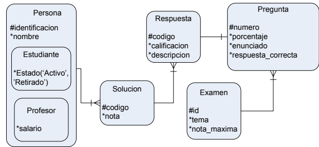
Figura 1. Diagrama entidad-relación de un sistema de notas en un colegio.
