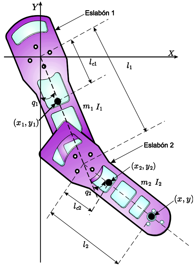
FIGURA 1. Robot rígido de dos grados de libertad.
