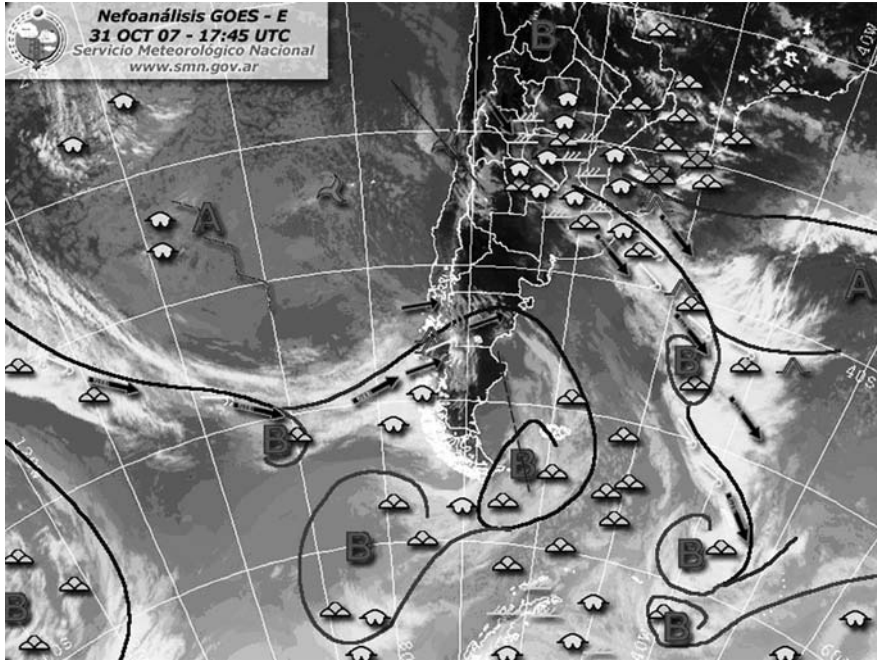
Figura 4. Carta sinóptica y neofanálisis del día 31 de octubre de 2007. Servicio Meteorológico Nacional ( www.smn.gov.ar ).
