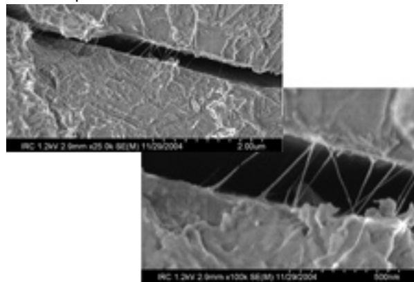
Figura 4. Nanotubos de carbono uniendo una grieta formada en el cemento [14].
