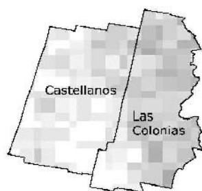
Figura 2. División de la superficie de los departamentos Castellanos y Las Colonias de acuerdo al nivel de endemidad para el Boophilus microplus utilizando el modelo de Estrada Peña (1999, 2001) como promedio del período 1989-2000. Mayor intensidad de gris indica mejor aptitud para la endemidad.
