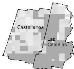
Figura 3. División de la superficie de los departamentos Castellanos y Las Colonias de acuerdo al mayor nivel de endemicidad para el Boophilus microplus utilizando el modelo de Estrada Peña (1999, 2001) para el período 1989-2000. Mayor intensidad de gris indica mejor aptitud para la endemicidad.
