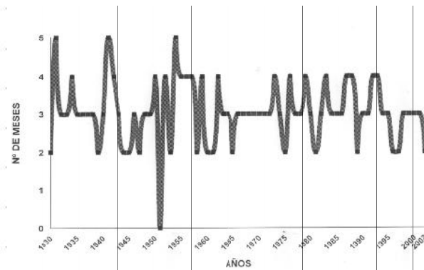
Figura 5. Número de meses con temperaturas promedio inferior a 15° C para la serie 1930-2002.
