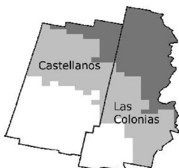
Figura 1. División de la superficie de los departamentos Castellanos y Las Colonias de acuerdo a los meses con temperatura promedio inferior a 15° C. Gris oscuro, gris claro y blanco indican 3, 4 ó 5 meses con temperaturas inferiores a ese valor. Programa LocClim 1.0 para el período 1960-1990.
