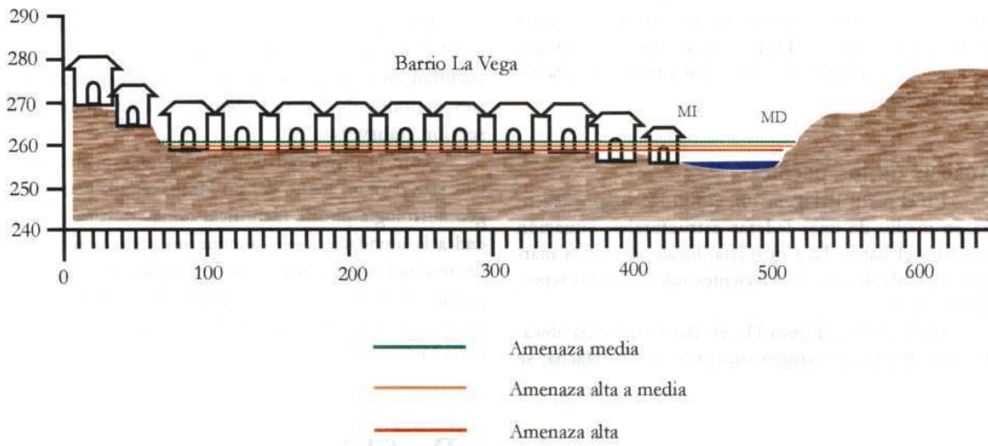
Figura 11. Perfil 2
