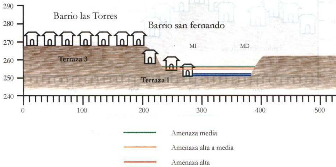
Figura 12. Perfil 3
