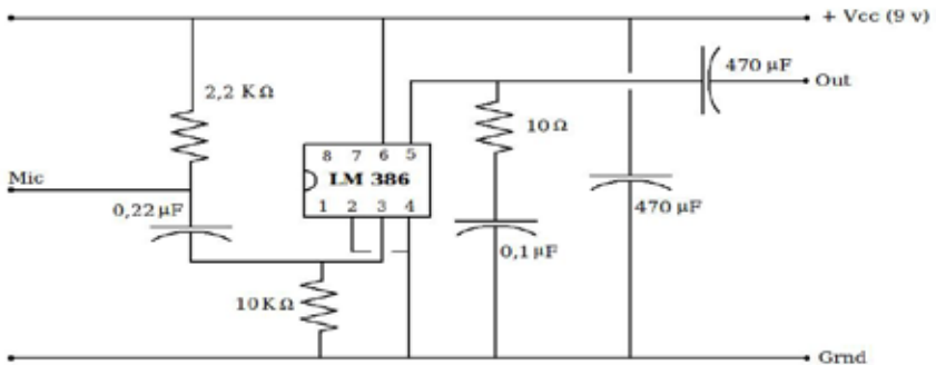
Figura 3. Circuito electrónico del amplificador de audio
