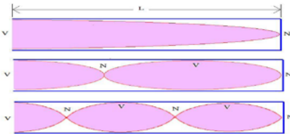
Figura 2. Los primeros tres armónicos que se forman dentro de un tubo con un extremo cerrado y el otro abierto
