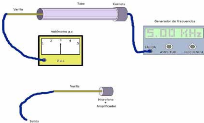
Figura 5. Montaje experimental
