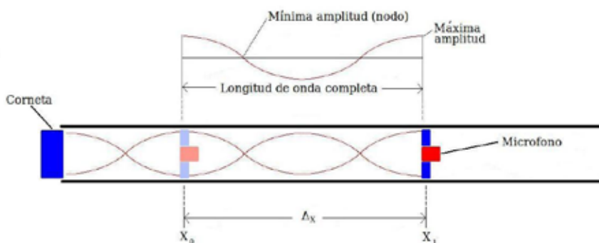
Figura 6. Formación de ondas dentro del tubo
