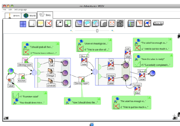
Figura 2. Interfaz de edición de narrativas de WEEV
