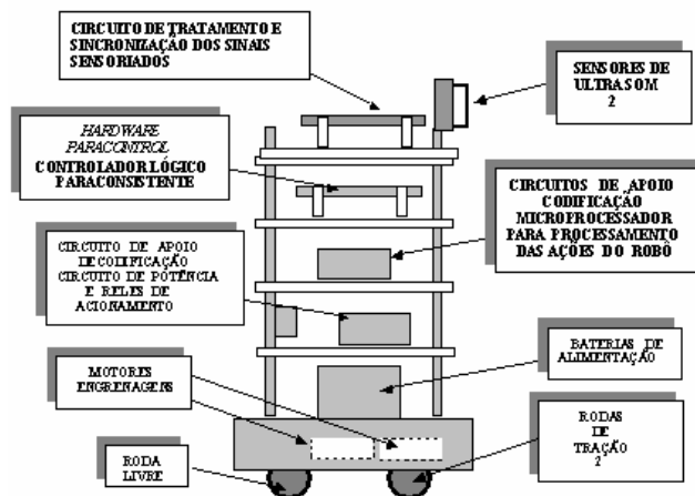
Figura 2 - Destaque das partes principais do robô Emmy
