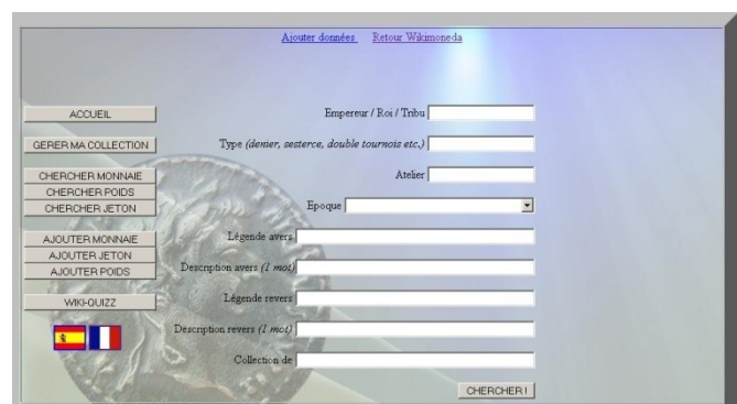
Figure 2 : Recherche avancée
