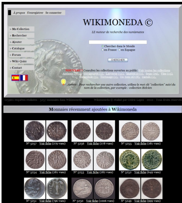
Figure 1 : Ecran d'accueil
