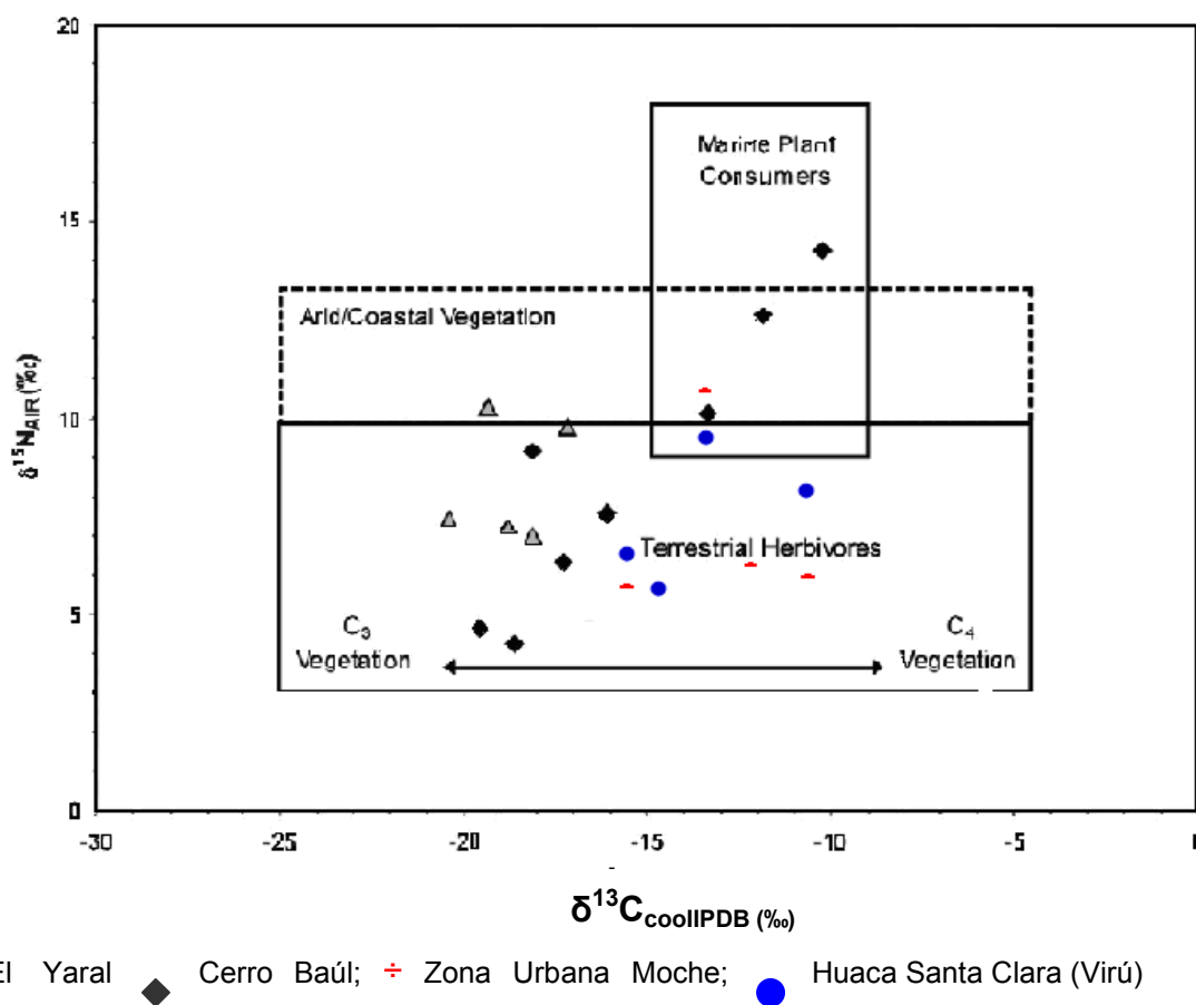
Figura 3. Valores de \delta^{13}C y \delta^{15}N obtenidos de colágeno de hueso de la Zona Urbana Moche, comparados con tres sitios costeros. Adaptado de Thornton et al (2011) y Szpak et al (2009).
