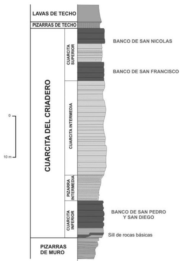
Figura 11. Columna estratigráfica esquemática de la Cuarcita del Criadero en la Mina de Almadén.
