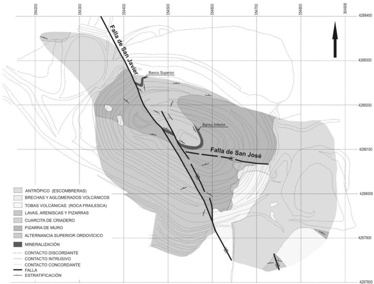
Figura 16. Esquema geológico de la corta de El Entredicho en los últimos momentos de la explotación. El mineral quedaba restringido al limbo de un sinclinal cortado por la falla transversal de San Javier.
