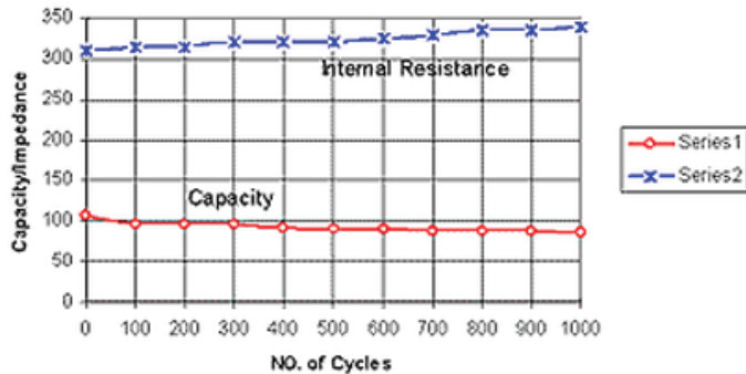
Fig. No. 5. Ciclo de rendimiento de iones de litio
