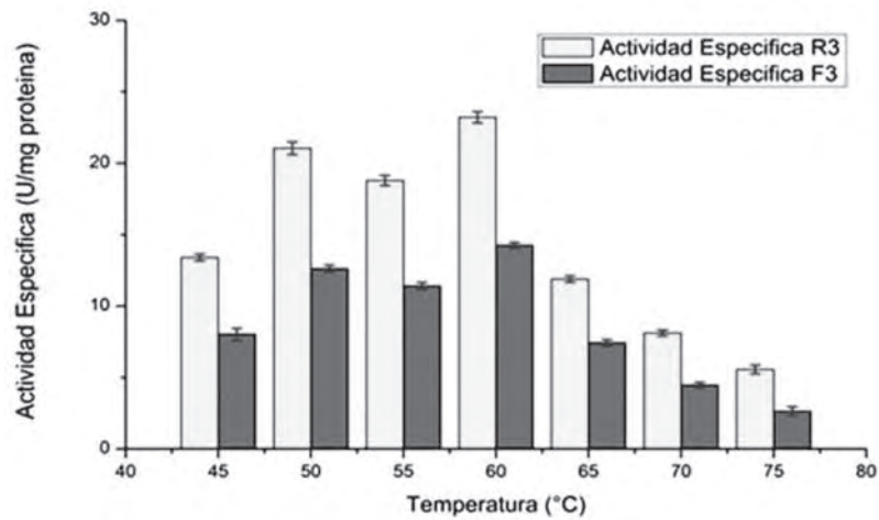
Figura 5. Actividad celulásica de extractos semipurificados de celulasas fracción R3 (>50 kDa) y F3 (<50 kDa) entre 45°C y 75°C.
