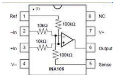
Fig. 7 Amplificador de instrumentación INA106
