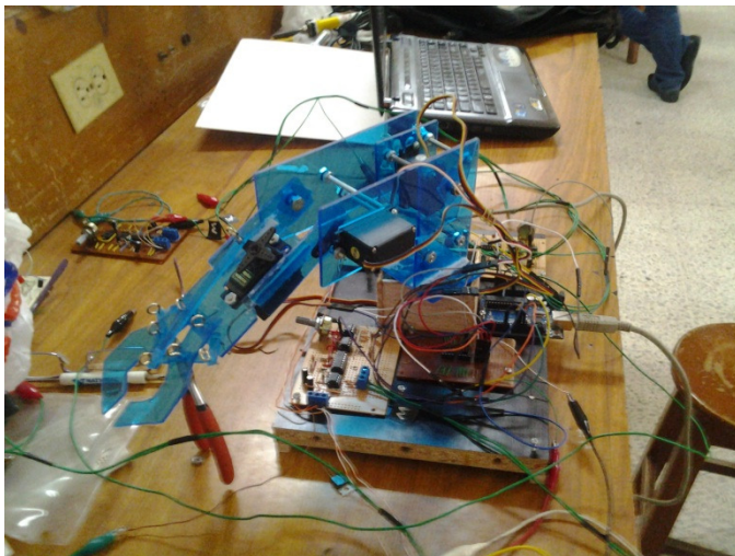
Fig. 12 Imagen del Brazo robótico
