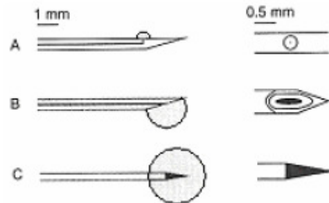
Fig. 2 Diferentes tipos de electrodos, A. Electrodo de fibra simple. B. Electrodo concéntrico. C. Electrodo monopolar [7].
