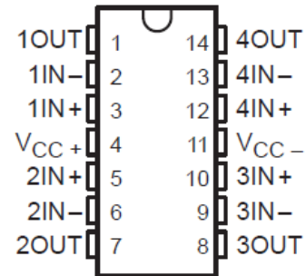
Fig. 8 Amplificador TL 074.
