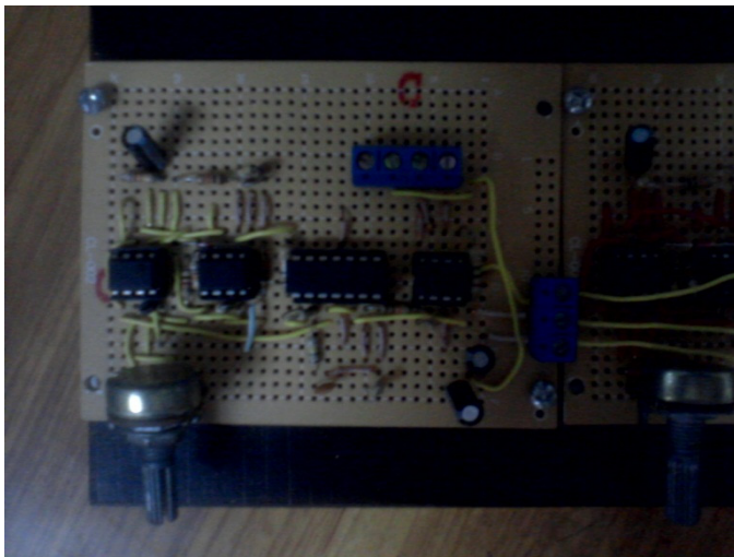
Fig. 11 Circuito en Baquela.
