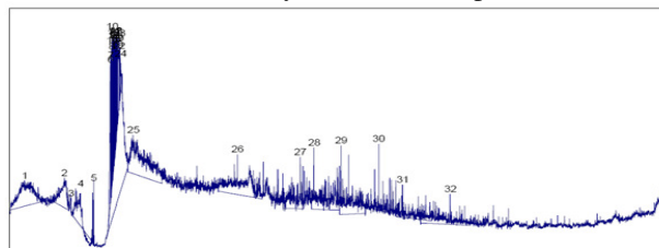
Figura 4. TIC del análisis por HPLC-ESI/MS de la fracción ODS-PF-1-2-C3. Sistema de elución gradiente de 10-60% CH 3 CN en 0.1% HCO 2 H por 80 min, con un flujo de 0.3 \mu L/min.
