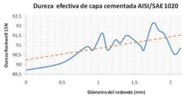
Fig. 3. Durezas de las probetas a) 8620, b) 1020
