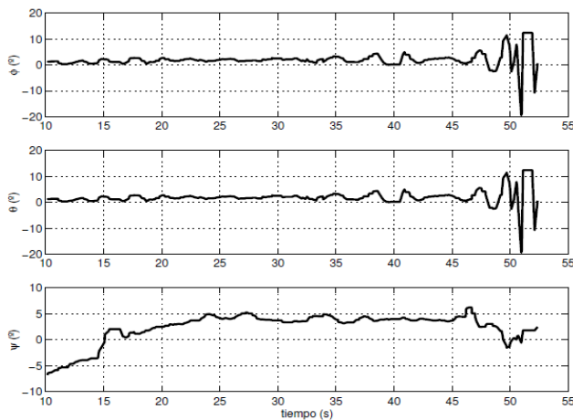
Figura 12: Orientación del helicóptero quadrotor.
