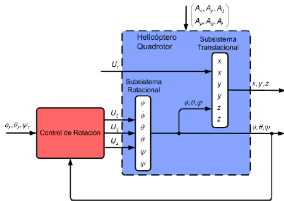
Figura 8: Control de orientación para el helicóptero quadrotor.
