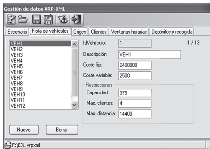
Figura 4. Configuración de restricciones.
