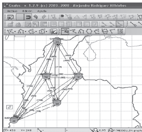
Figura 3. Esquema de los nodos del problema.
