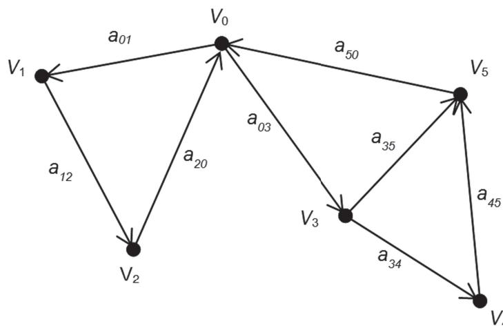
Figura 1. Representación esquemática de un grafo dirigido
