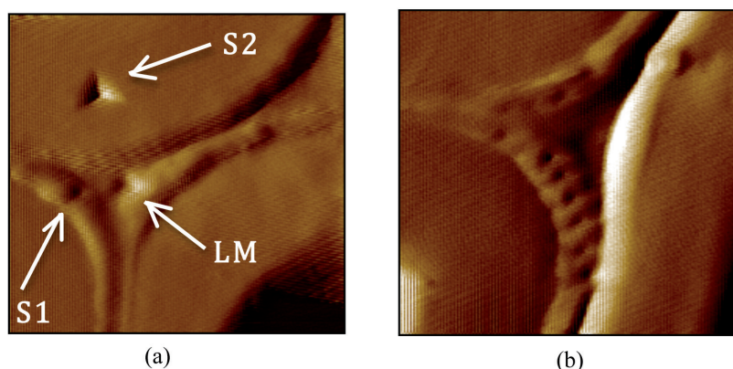
Figura 1. Imagen de nanoindentaciones en familias de Eucalyptus nitens . (a) En la lamela media (LM), y las capas S1 y S2, (área de escaneo: 5 \times 5 \text{ }\mu\text{m}^2 ). (b) En capa S1, (área escaneo: 4 \times 4 \text{ }\mu\text{m}^2 ).
