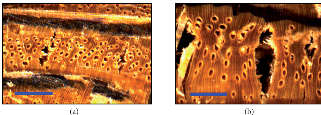
Figura 2. Imagen de microgrietas y vasos en familias de Eucalyptus nitens . (a) Anillo de crecimiento 6, sitio de Mulchén. (b) Anillo de crecimiento 7, sitio de Yungay.
