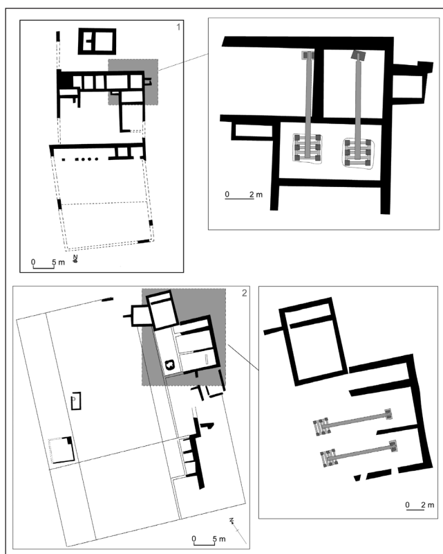
Figura 3. Instalaciones de prensado: 1, El Moré; 2, Veral de Vallmora (según Martín Olivares – Bayés, 2009; tratamiento informático M. Cubero).
