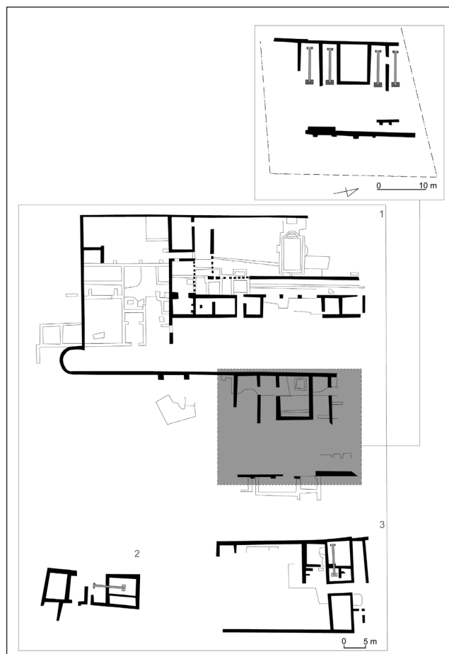
Figura 5. Instalaciones de prensado y hábitat rural: el ejemplo de la villa dels Ametllers (1) y los asentamientos secundarios de Ses Alzines (2) y Mas Carbotí (3), en el litoral del Tosa de Mar (según Palahí – Nolla, 2010; tratamiento informático M. Cubero).
