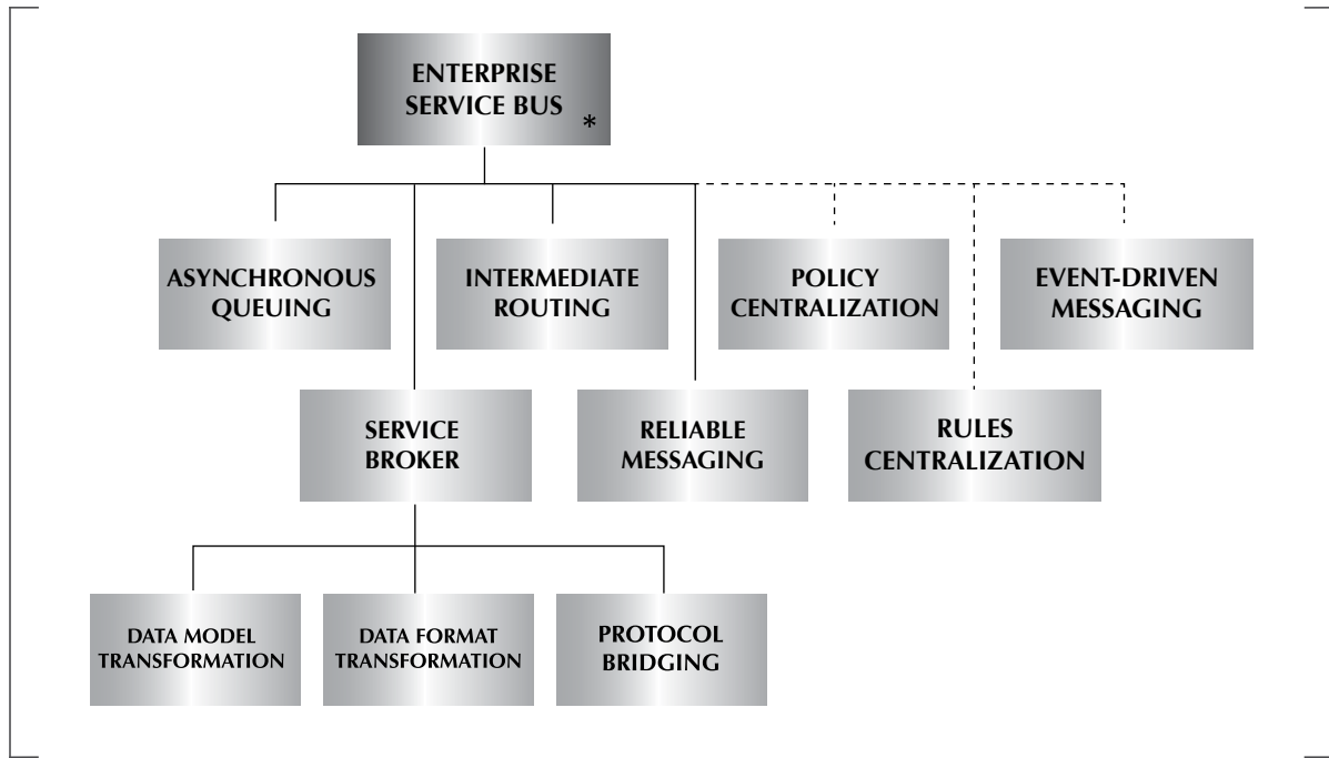
Figure 14. Enterprise service bus (Erl, 2008b)
