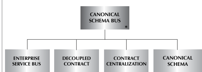
Figure 13. Canonical Schema Bus (Erl, 2008b)
