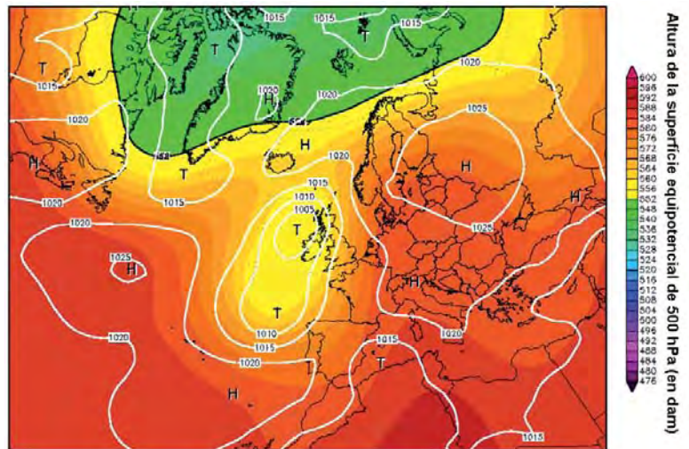
Figura 18. Altura en decàmetres de la superfície equipotencial de 500 hPa (en taques de color) i isòbares de pressió atmosfèrica en superfície en hectopascals (línies blanques) a les dotze de la nit del dia 23 de setembre de 1874. Els colors taronja sobre la Mediterrània occidental indiquen la presència d'una massa d'aire càlid a uns 5.500 m d'altura (que uns dies abans es trobava sobre Catalunya) i la lletra T sobre les illes Balears indica la presència d'una depressió. Font: Wetterzentrale.de.
