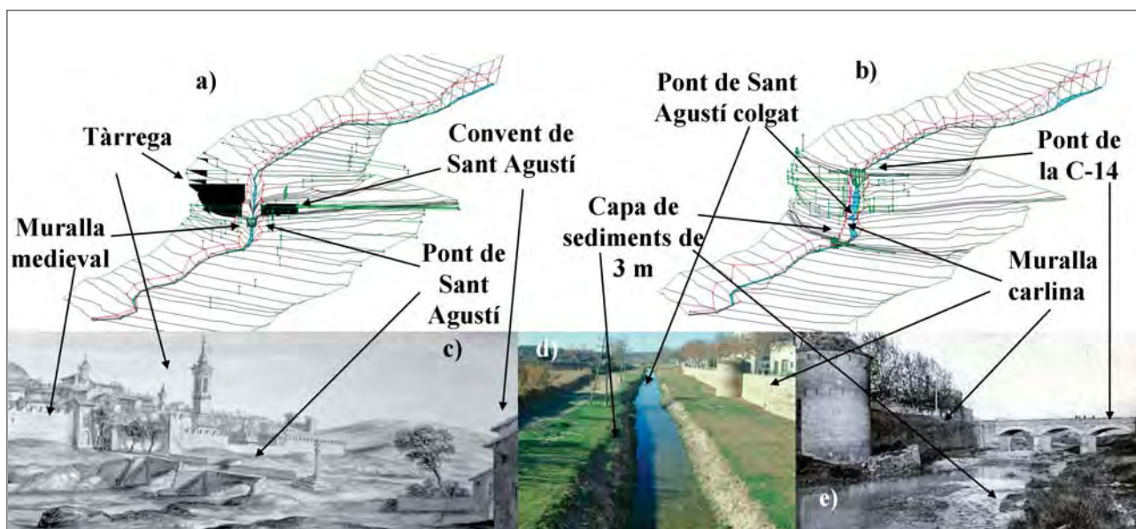
Figura 11. Geometria del tram del riu Ondara al seu pas per Tàrrrega i els obstacles al flux a) abans i b) després de la modificació causada per la deposició de sediments; c) dibuix de Pier Maria Baldi, del 1668; d) vista del tram mirant aigües amunt amb el pont de la C-14; e) vista del tram aigües amunt, amb el pont de la C-14 al fons. Font: elaboració pròpia.
