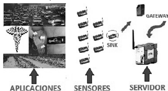
FIGURA 1. Arquitectura WSN.
