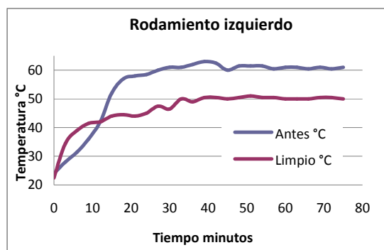
Grafica 3: Comparación rodamiento izquierdo de la zaranda antes y después de la limpieza.
