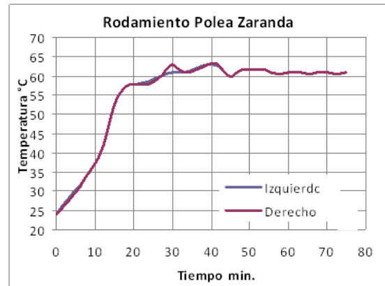
Grafica 1: comportamiento de la temperatura en el rodamiento derecho.
