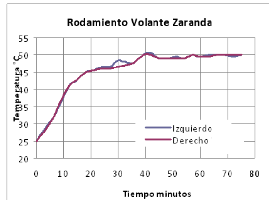
Grafica 2: comportamiento de la temperatura en el rodamiento izquierdo de la zaranda
