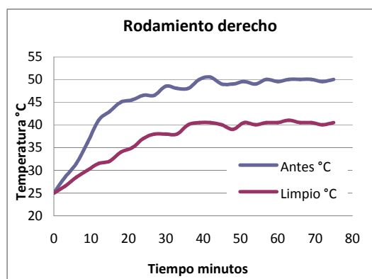
Grafica 4: Comparación rodamiento derecho de la zaranda antes y después de la limpieza.
