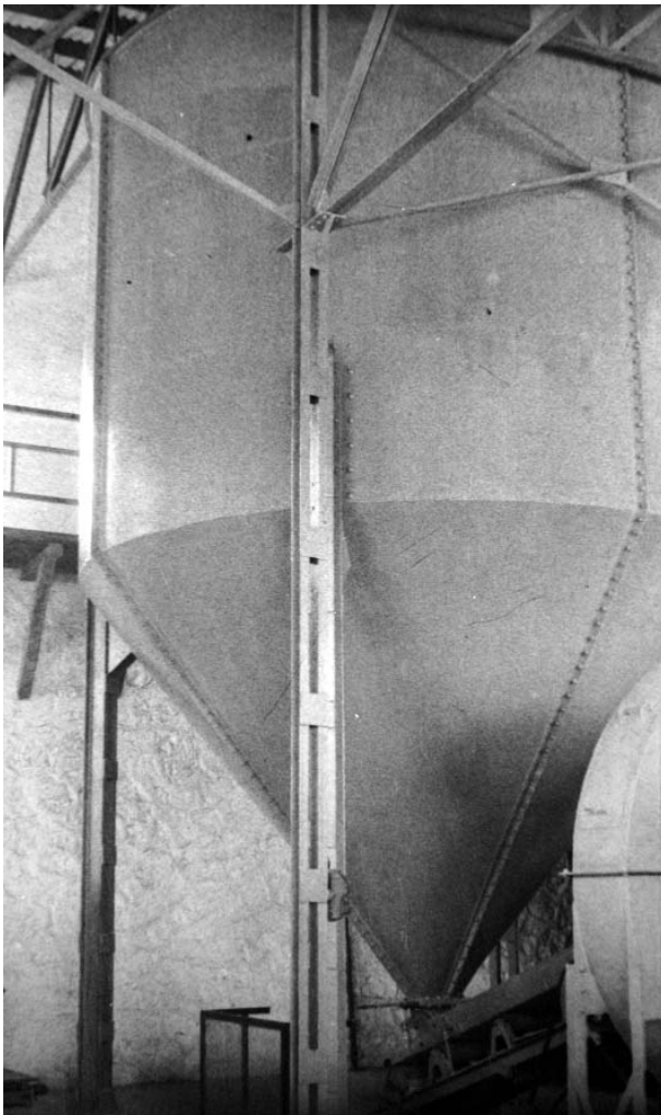
Figura 10. Tolva de menudo (Bou Mon, 1952).
