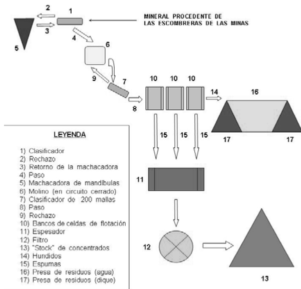
Figura 15. Esquema simplificado de planta metalúrgica por flotación del rincón de Martos de la empresa TRAMISA (década de los años 1950), Sierra del Cabo de Gata (Almería) (elaboración propia; sin escala).
