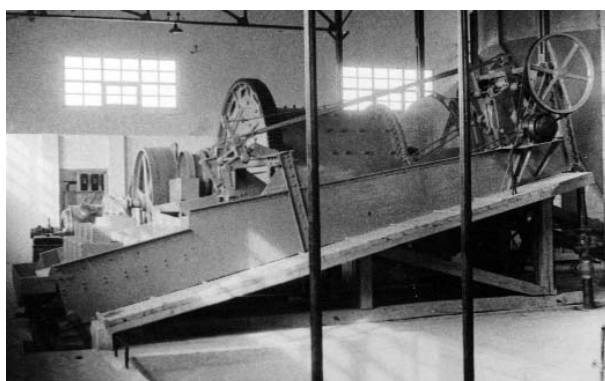
Figura 8. Clasificador Dorr (Bou Mon, 1952).
