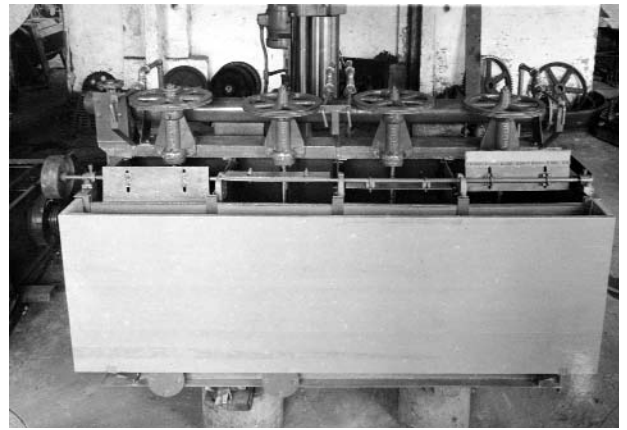
Figura 12. Máquina de flotación número 2 (Martín Pérez, 1950).
