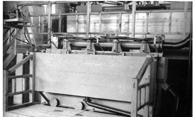
Figura 13. Banco de celdas de flotación del lavadero (Bou Mon, 1952).
