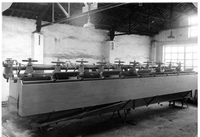
Figura 17. Banco de celdas de flotación (Martín Pérez, 1950).
