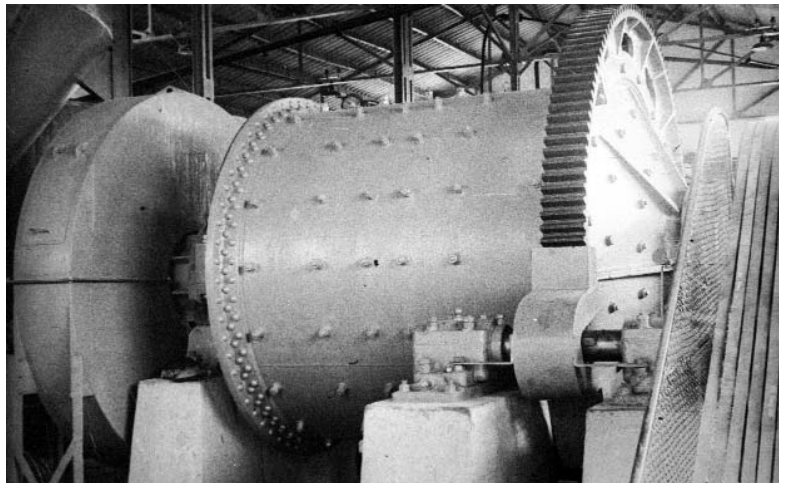
Figura 16. Molino de bolas utilizado en la fase de molienda (Bou Mon, 1952).
