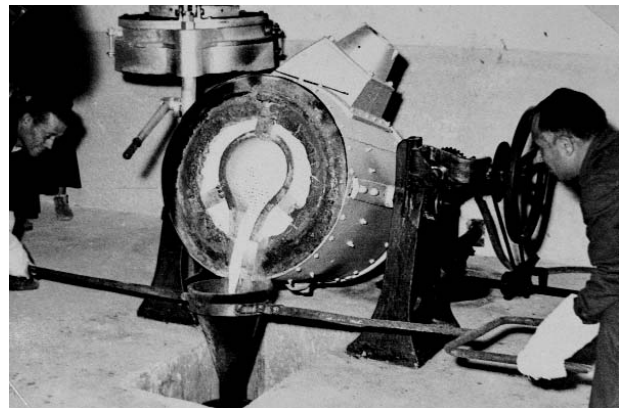
Figura 24. Proceso de fundición de un lingote de oro (Fernández Espinar, 1958).
