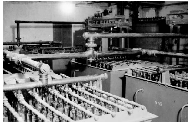
Figura 22. Celdas de precipitación de la casa P.A.F. (Fernández Espinar, 1958).
