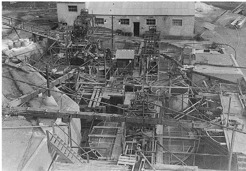
Figura 14. Zona de agitación y de lavado contracorriente (Morales López, 1936).
