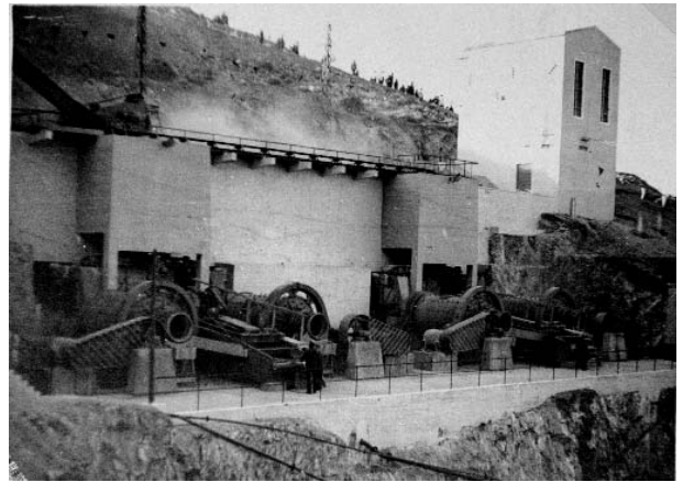
Figura 21. Zona de molienda en húmedo (Fernández Espinar, 1958).
