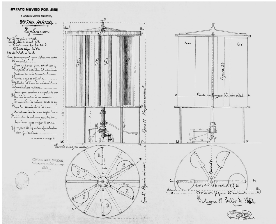
FIGURA 1: Sistema Bartual. Expediente de patente n.º 4409. AHOEPM
