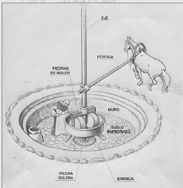
ESQUEMA DEL MOLINO DE CACAO DE CORIAS 5
