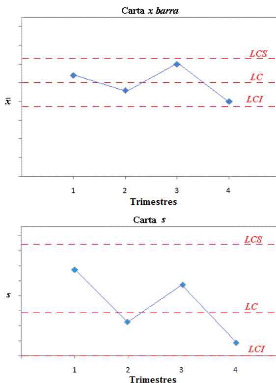
Figura 1. Cartas de Control x barra – s para el Laboratorio de Metrología de Variables Eléctricas de la UTP
