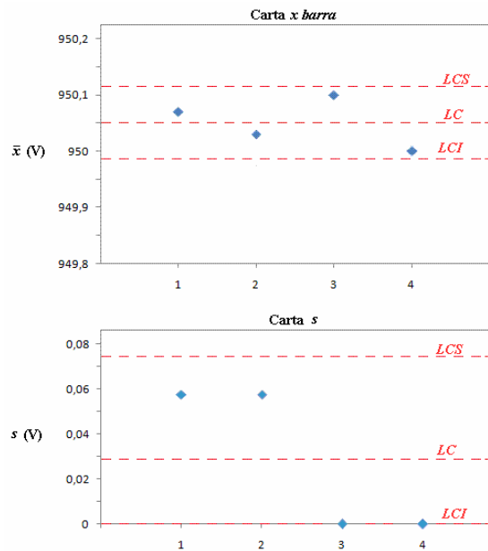
Figura 2. Cartas de Control x barra – s para los Datos del Ejemplo
