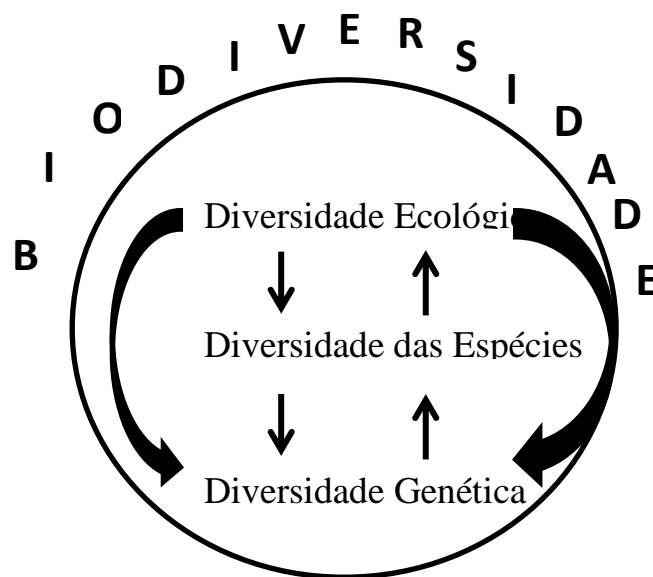
Figura 1: O conceito de biodiversidade aplica-se ao conjunto da diversidade ecológica, diversidade de espécies e diversidade genética, assim como à sua interação (Adaptado de BARBAULT, 1998).
