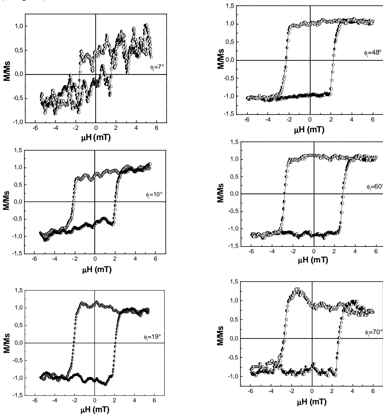
Figura 2. Ciclos de histéresis para diferentes ángulos de incidencia del haz lumínico en el magnetómetro Kerr.
