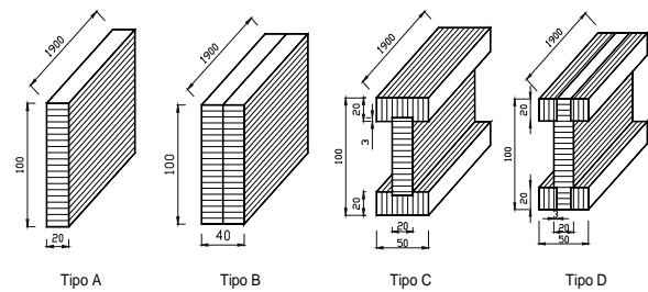
Figura No. 1 Tipo de sección vigas laminadas de guadua angustifolia Kunth.
