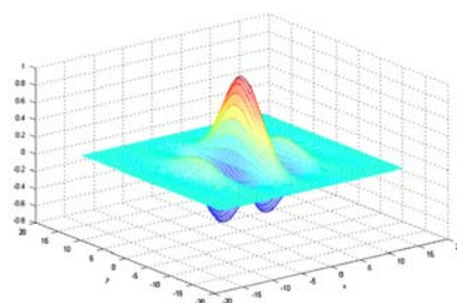
Figura 5. Ejemplo de una función base de Gabor para 2D.
