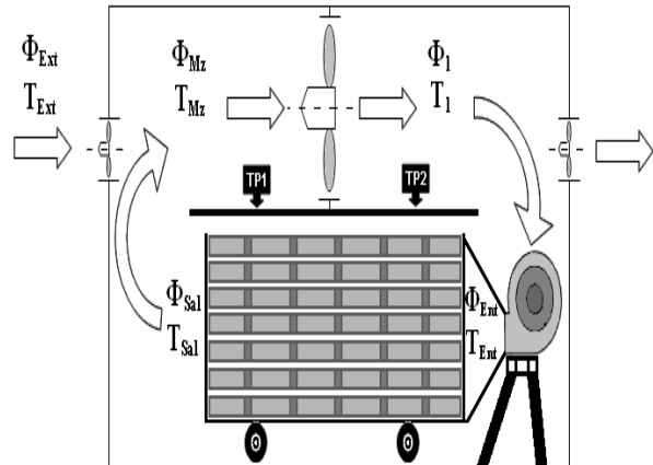
Fuente: Autor Figura 6. Zonas establecidas de temperaturas y humedades en la prueba de secado con ventilación axial y ventilación centrífuga forzada
