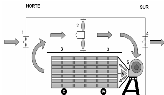
Figura 2. Esquema de circulación de aire caliente con ventilación axial y ventilación centrífuga forzada
