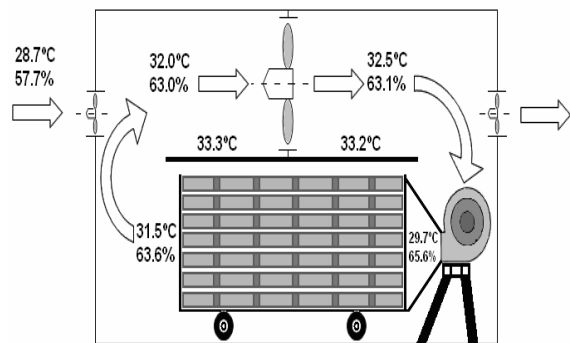
Fuente: Autor Figura 7. Valores promedio de Humedades y Temperaturas correspondientes a las zonas establecidas en la prueba de secado con ventilación axial y ventilación centrífuga forzada
