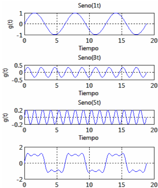
Figura 1. Señal Cuadrada con seis coeficientes
