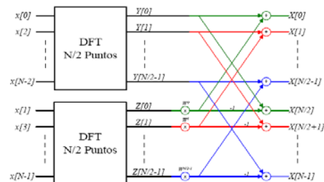
Figura 3. Diagrama Mariposa del Algoritmo de 4 puntos
