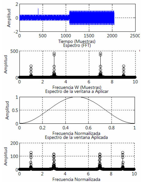
Figura 5. Análisis de una señal no estacionaria con FFT.
