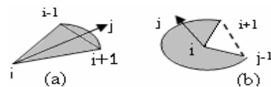
Figura 8 La diagonal s = ij esta en el cono determinando por v_{i-1} , v_i v_{i+1} : figura 8 (a) convexo y la figura 8. (b) reflejo. En (b) ambos v_{i-1} y v_{i+1} esta a la derecha de ij .
