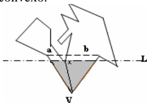
Figura 3. vx puede ser una diagonal
