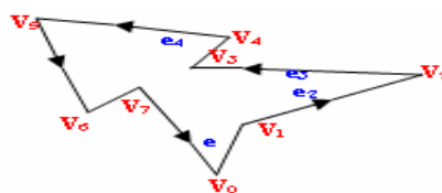
Figura 1. Polígono con vértices orientados en sentido antihorario.
