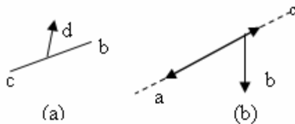
Figura 7. (a) Intersección Impropia entre Segmentos. (b) La Colinealidad no es suficiente.
