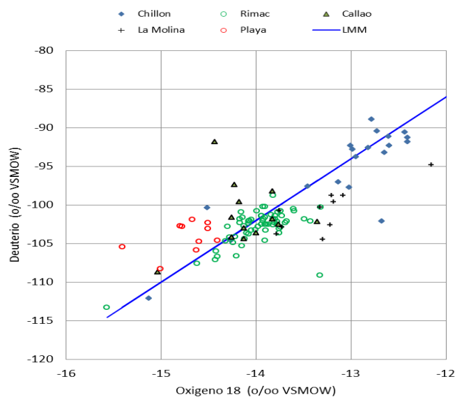
Fig. 1: Isotopos estables de aguas del acuífero de Lima y de manantiales de la Costa Verde
