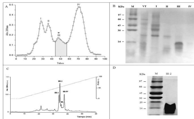
Figuras 1: A) Cromatografía de exclusión molecular en Sephadex G-75 del veneno bruto de Micrurus spixii . B) Gel de SDS-PAGE con las muestras de la cromatografía de exclusión molecular en columna de Sephadex G-75, veneno total (VT) y fracciones de Micrurus spixii , I, II, III y IV. Siendo M el marcador molecular. C) Cromatografía en sistema HPLC-fase reversa en una columna analítica C-18 µ-Bondapak (Waters) del pico III de Sephadex G-75. D) Gel de SDS-PAGE con las muestras da cromatografía en HPLC de fase reversa, marcador y III-2 fracción obtenida de la cromatografía en HPLC de fase reversa.
