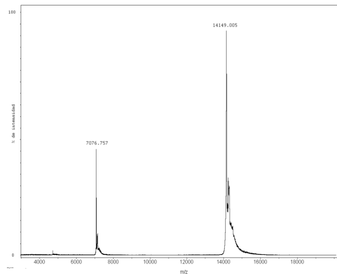
Figura 2. Espectro de masa molecular de la fracción III-2 procedente del veneno de Micrurus spixii
