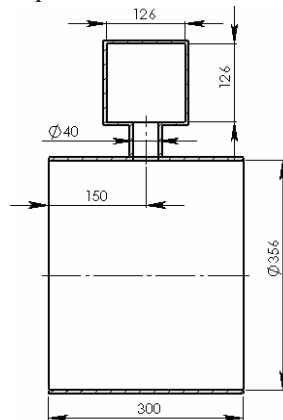
Figura 8. Resonador de Helmholtz instalado en el ducto, dimensiones en milímetros.
