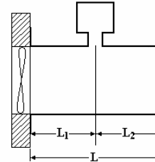
Figura 2. Resonador de Helmholtz instalado en un ducto de longitud finita
