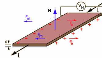
Figura 1. Sensor de Efecto Hall
