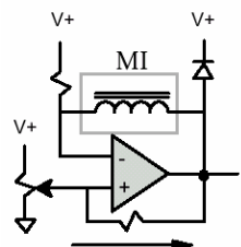
Figura 5. Sensor MAGNETOINDUCTIVO
