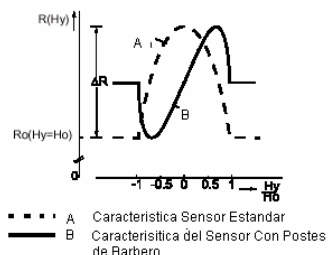
Figura 3. Curvas características del sensor magnetoresistente
