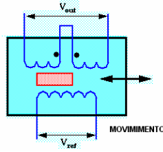
Figura 6. Sensor con Transformador de Corriente
