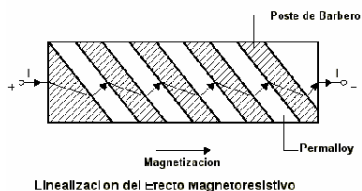
Figura 4. Linealización del efecto Magnetoresistivo
