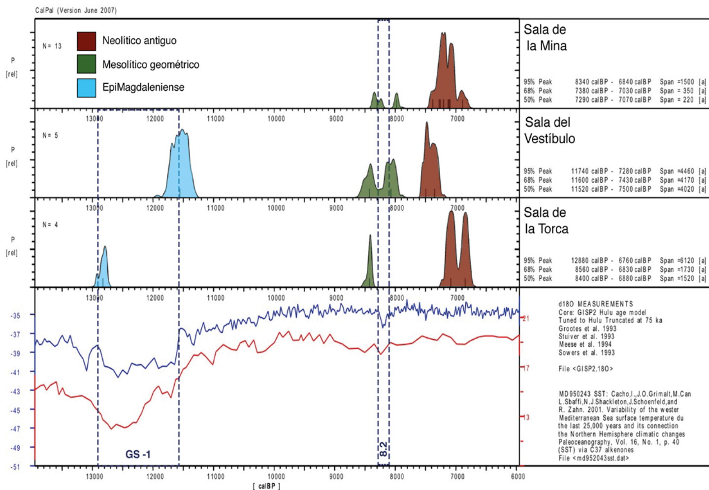
Fig. 4: Cueva de Nerja. Curvas de probabilidad acumulada obtenidas a partir de la calibración de las fechas de la Tabla 1 (Weninger et al. , [2007], comparadas con 2 proxies de alta resolución: GISP2 (variación ^{18}\text{O} / \text{O}^{16} ) (Grootes et al. , 1993; Meese et al. , 1994; Sowers et al. , 1993) y SST del mar de Alborán (Cacho et al. , 2001).
