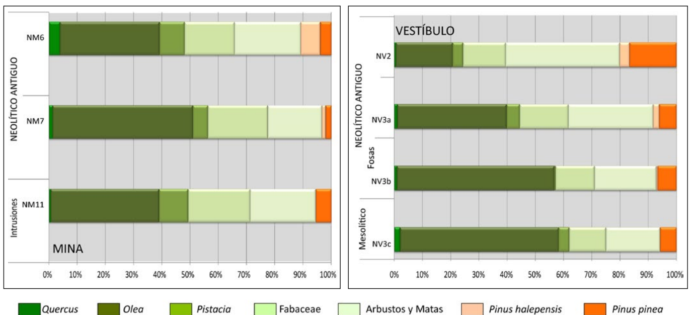
Fig. 3. Cueva de Nerja: vegetación leñosa identificada en los niveles arqueológicos holocenos con una cantidad de carbón suficientemente representativa.
