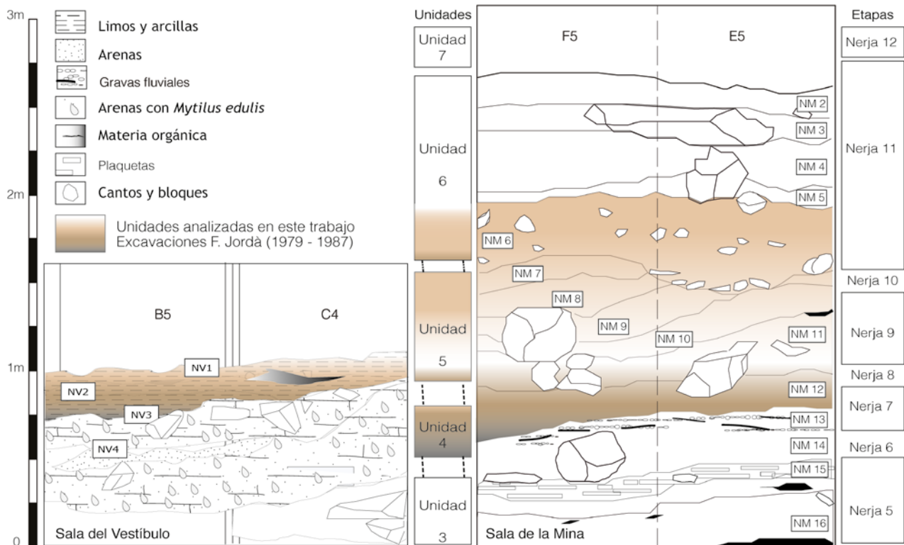
Fig. 2. Cueva de Nerja. Planimetría de las salas con indicación de la procedencia de los materiales y correlación litoestratigráfica del tramo estudiado en las salas de la Mina y del Vestibulo.
