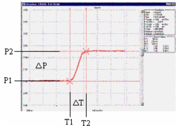
Figura 5. Incremento de presión en la manguera
