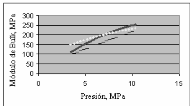
Figura 6. Módulo de bulk efectivo. ----- 1 metro, — 2 metros, .....3 metros.
