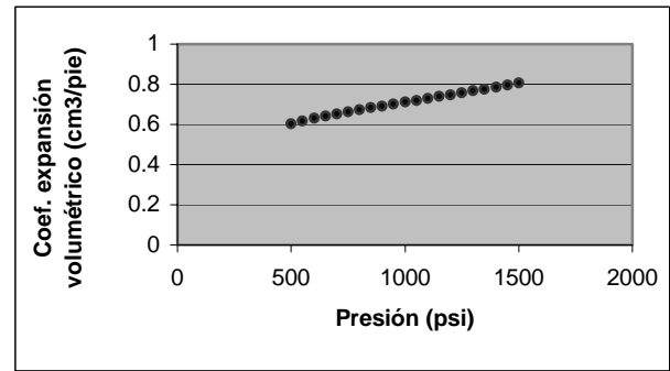
Figura 8. Coeficientes de expansión volumétrica para mangueras tipo 100R2 AT -06.
