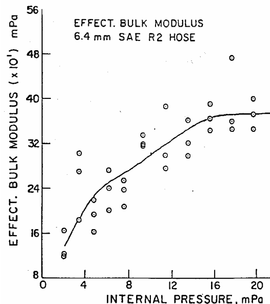
Figura 9. Módulo de Bulk efectivo para manguera SAE R2
