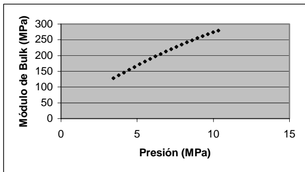
Figura 7. Módulo de bulk. Manguera tipo 100R2 AT -06.
