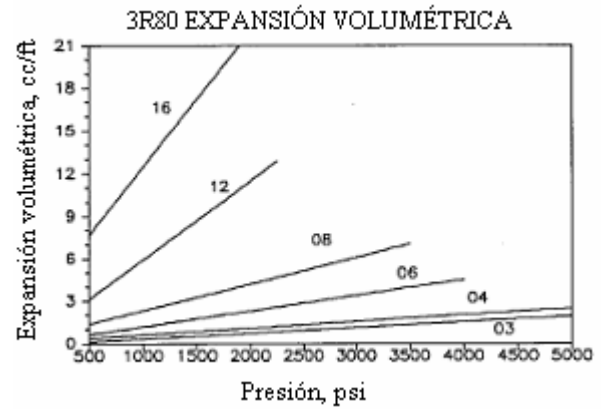
Figura 3. Coeficiente de expansión volumétrica Vs presión para mangueras tipo SAE 100R8 de diferente tamaño [6]
