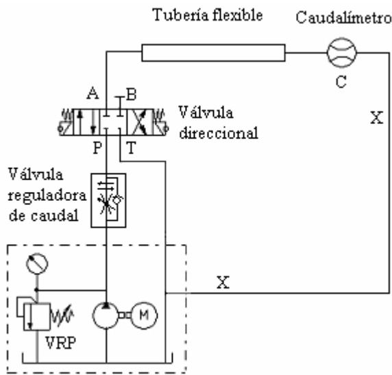
Figura 4. Circuito hidráulico utilizado para determinar el módulo de Bulk efectivo.
