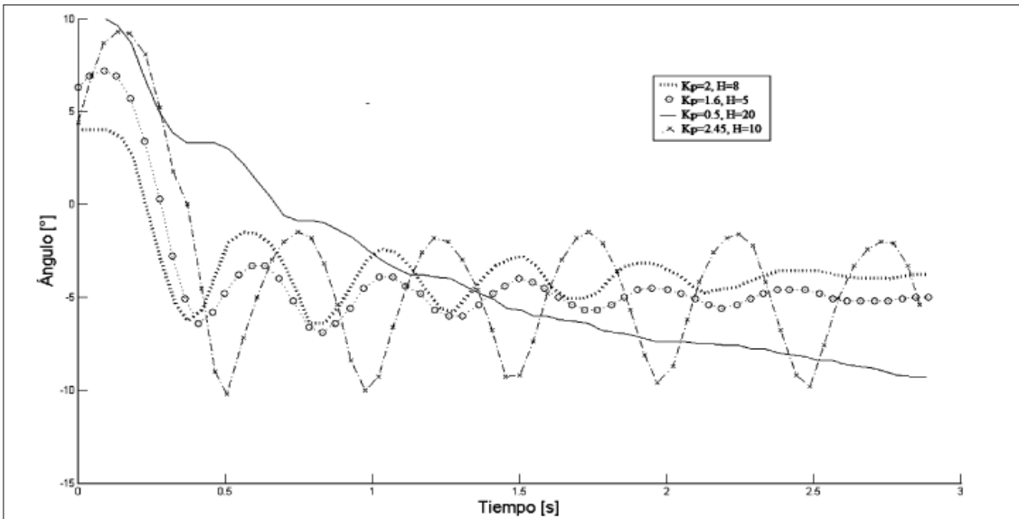
Figura 6. Respuesta del sistema frente a un escalón de bajada
