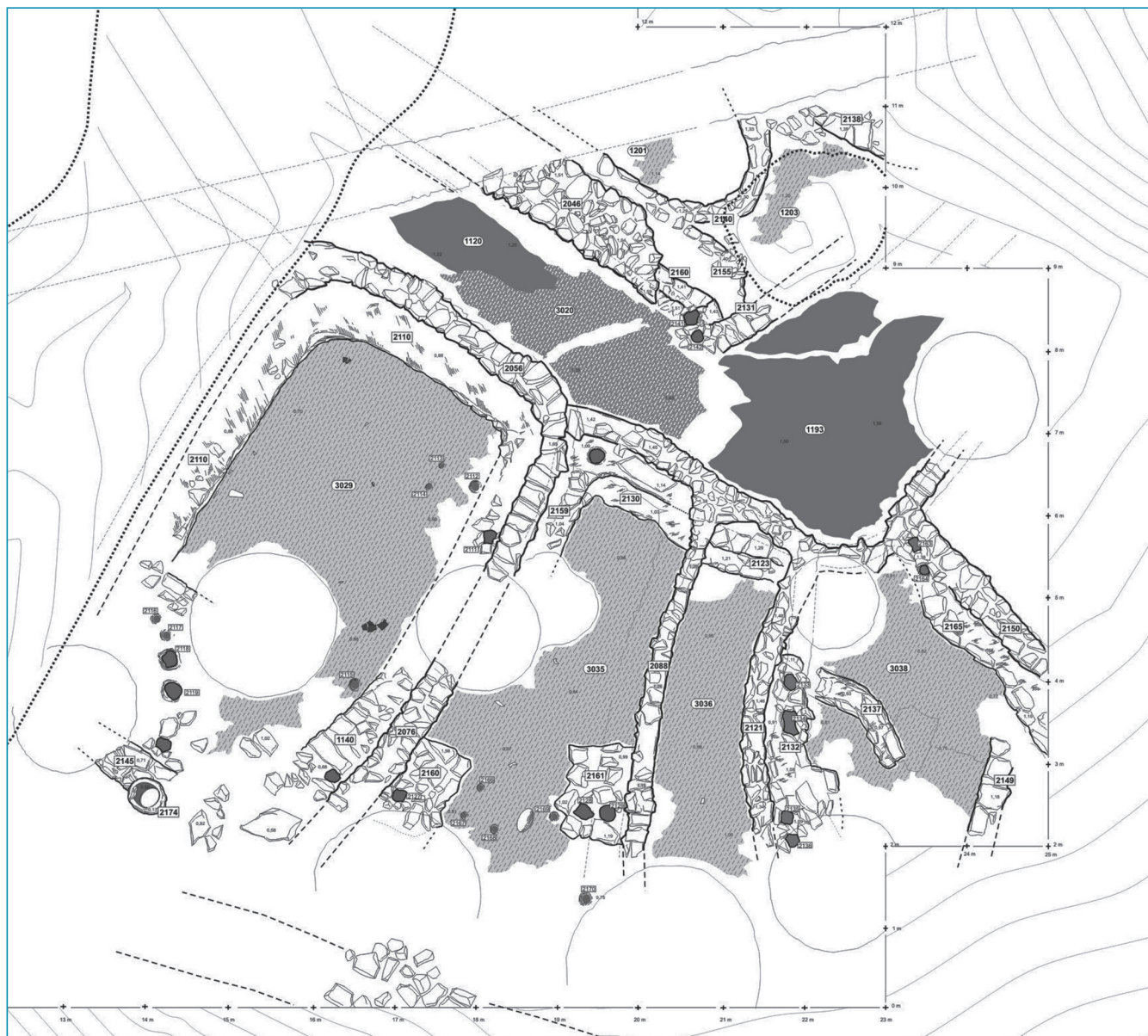
Figura 2. Cabezo Pardo. Planta general del Sector 2 con las estructuras y pavimentos registrados correspondientes a la Fase II del asentamiento argárico (1800-1650 cal ANE, aprox.)
