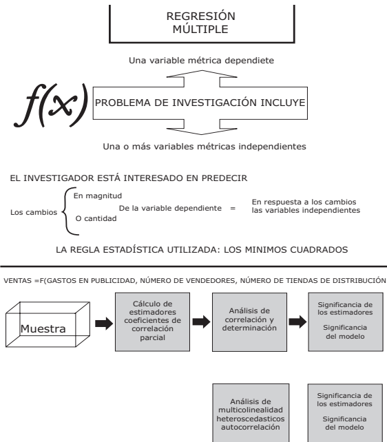
Figura 10c. Regresión múltiple
