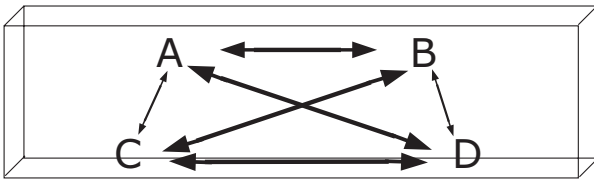
Figura 12c. Escalamiento multidimensional
