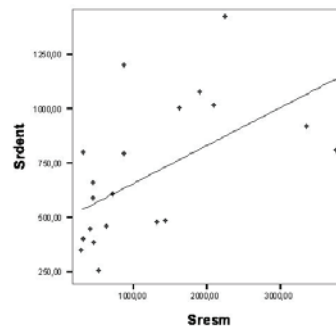
Figura. 2.- Gráfica que muestra la relación entre el estroncio de la dentina y del esmalte.
