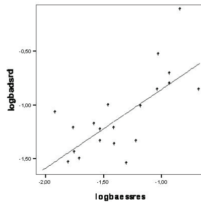
Figura. 1.- Gráfica que muestra la relación entre el logaritmo Ba/Sr en dentina y esmalte.
