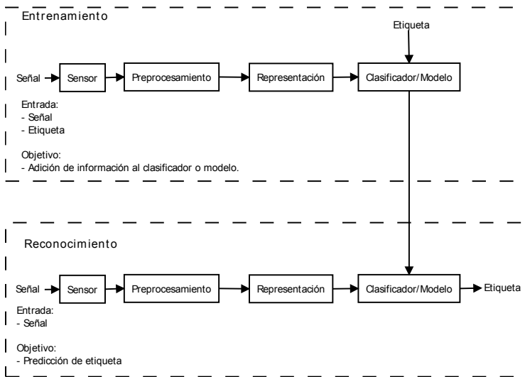
Figura 1: Etapas de un sistema de reconocimiento. El sistema se divide en entrenamiento (arriba) y reconocimiento (abajo). En cada una de estas partes se encuentran las etapas de adquisición, preprocesamiento, representación y clasificación.
